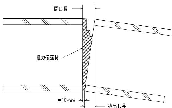
継手部開口長
