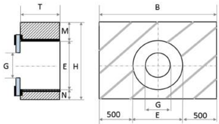
発進坑口標準寸法図
