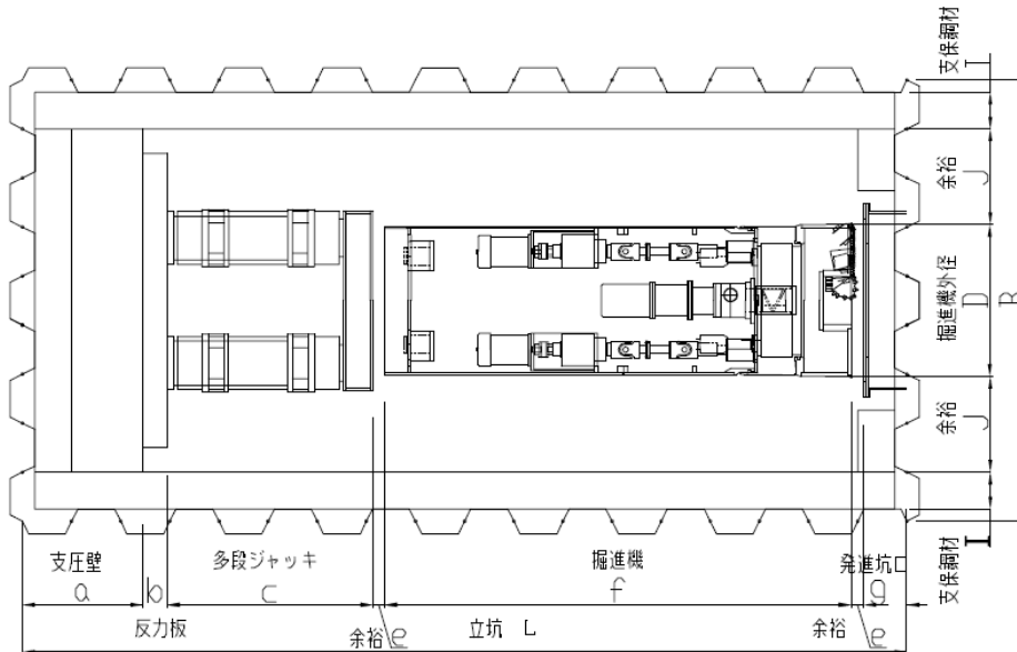
発進立坑（平面図）
