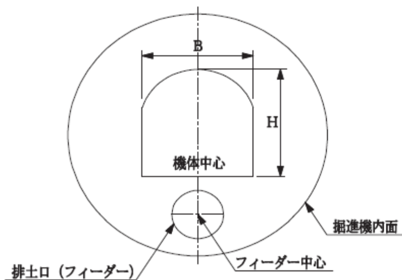
点検扉標準図
