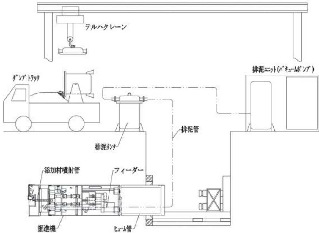
吸引排土システムのフローシート
