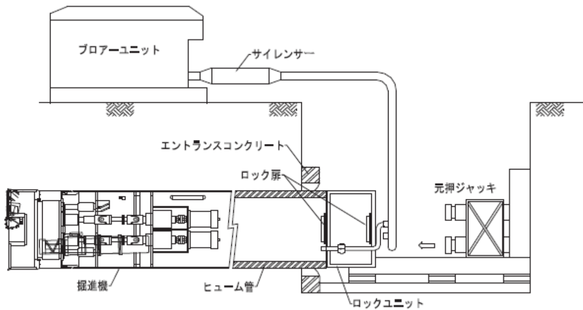
圧気工法のフローシート
