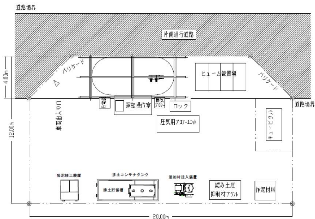
吸引排土方式坑外設備配置例 約 240m 2
