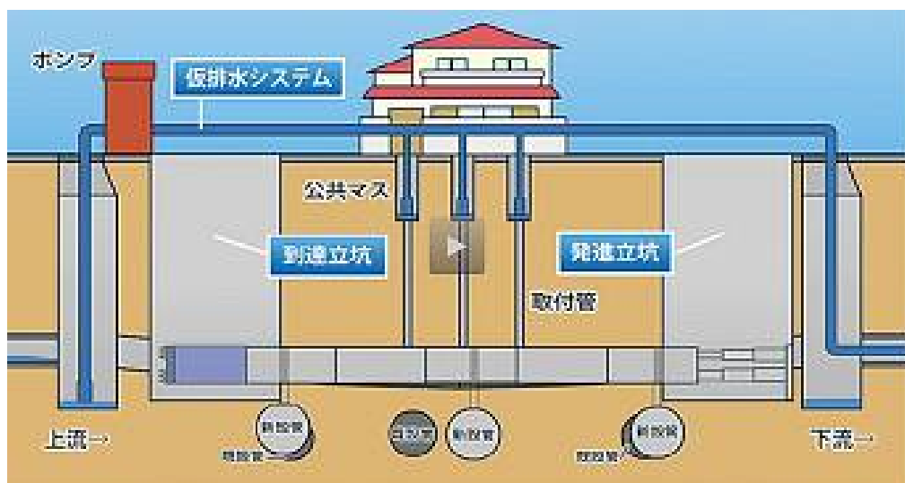
仮排水システム
